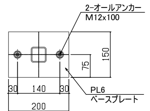
BPL詳細図
