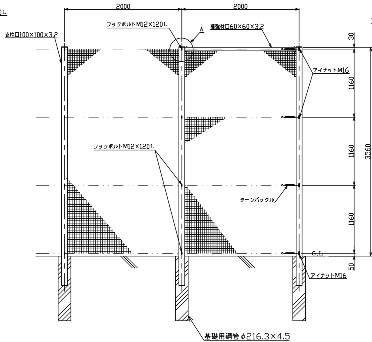
立面図 S=1:40
