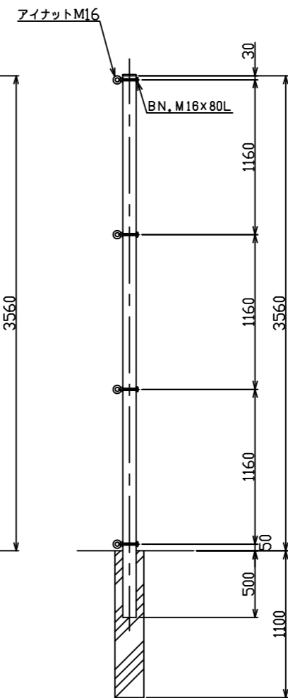
側面図 (端末) S=1:40
