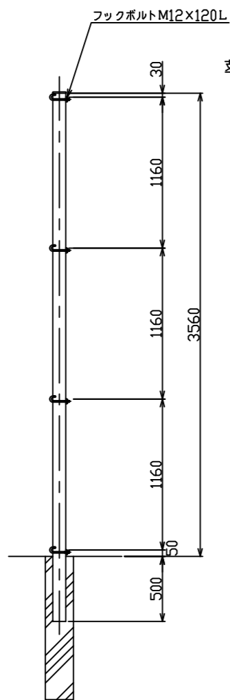
側面図 (中間) S=1:40
