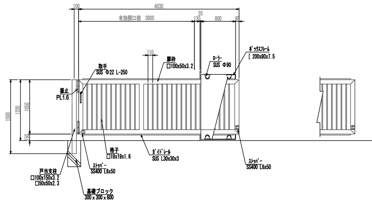
正面図
