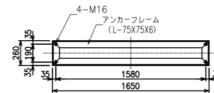
アンカーフレーム詳細図
